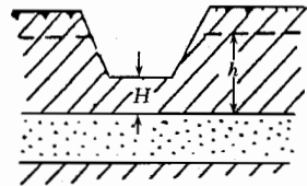
图 7.1 含水层示意图
