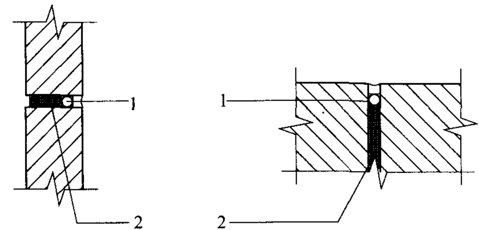
图 6.5.7 控制缝构造
