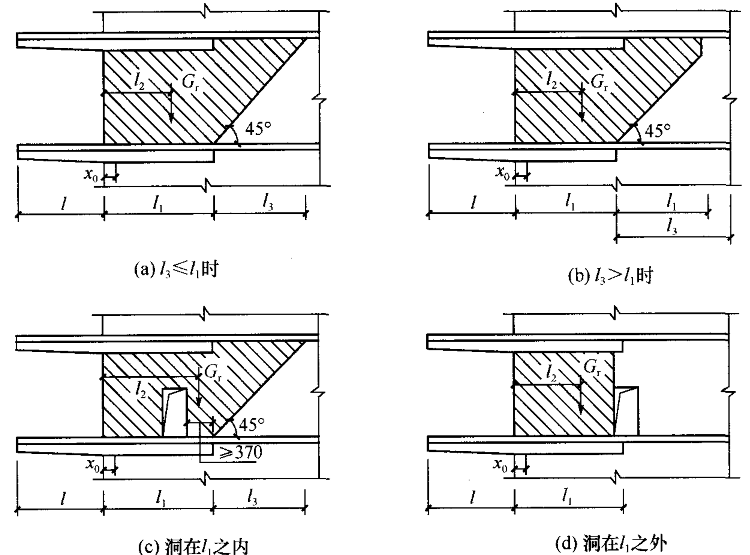
图 7.4.3 挑梁的抗倾覆荷载
